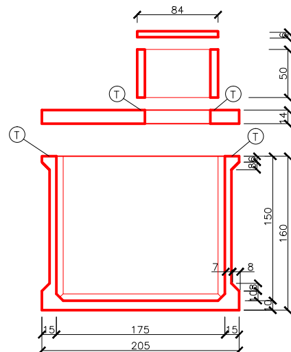
ŘEZ C-C'
