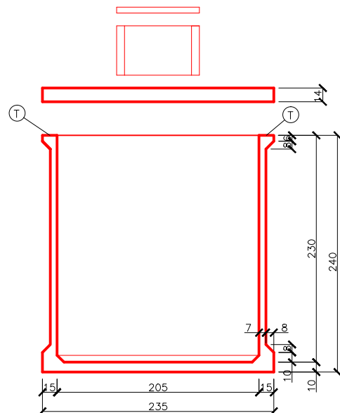
ŘEZ C-C'
