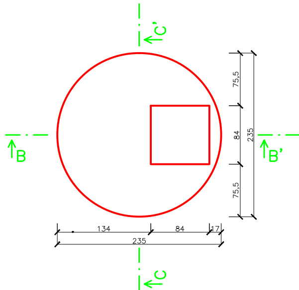
PUDORYS
