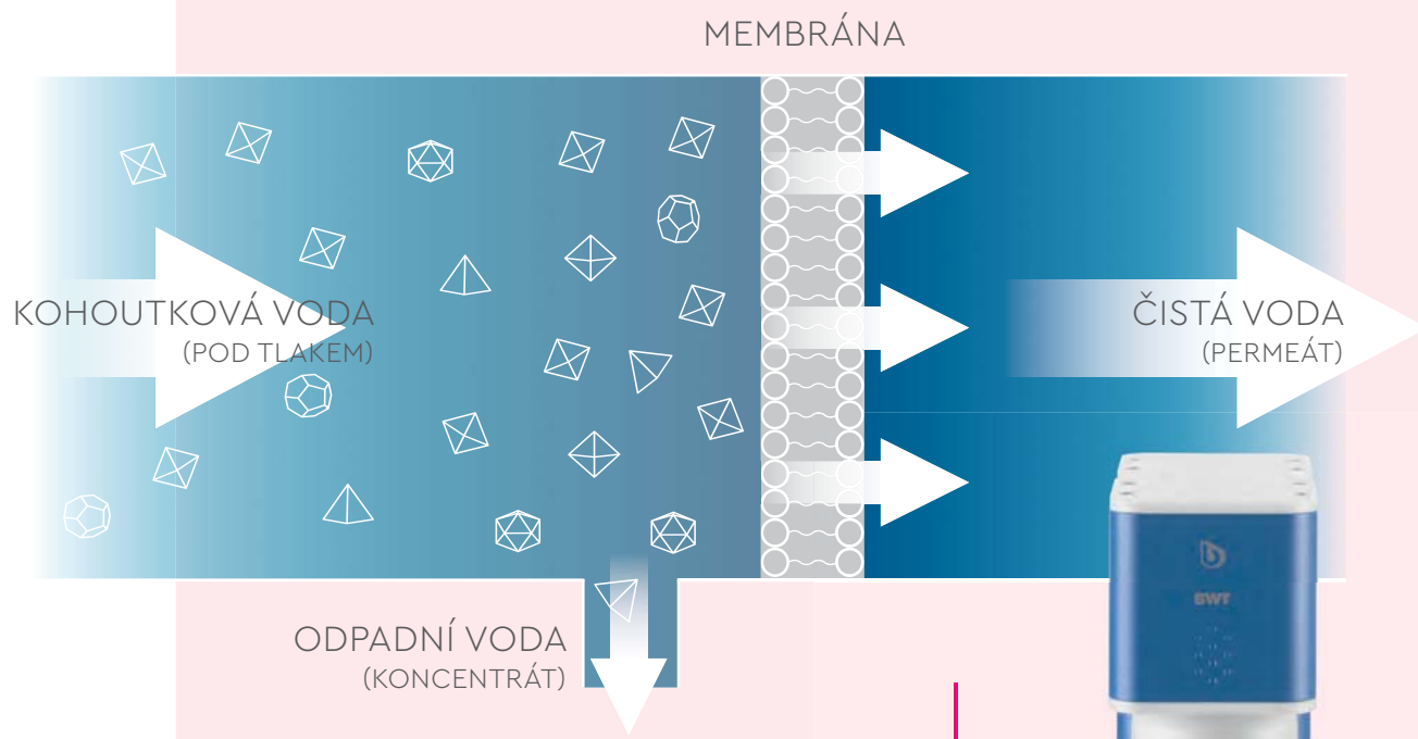
Schéma reverzní osmózy (separační proces)
