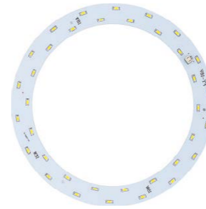
6574 LED MODULE Ø 25cm 18W 1800lm, 4000K
