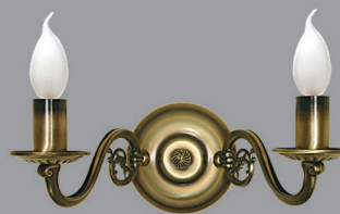
381/K2 ↔ 30 cm ↔ 20 cm $25 cm 2 x E14 max 60 W
