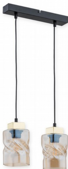
O2962 W2 CZA + ZL 2 x E27 max 60 W H 30 - 70 cm · W 32 cm · D 11,5 cm
