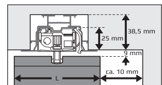
Anbringung mit Sonderzubehör Einbauprofil. (Schienenbefestigung mit Kunststoffclip.)
