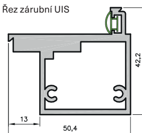
Řez zárubně UIS
