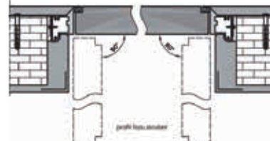
Řez zárubně UIS
