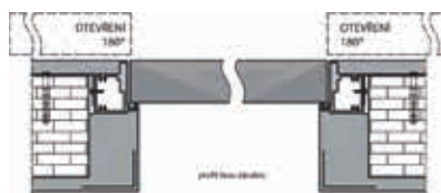
BEZFALCOVÉ KŘÍDLO OTEVÍRAVÉ VEN
