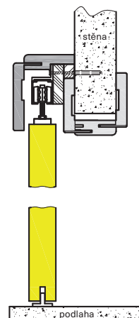
Posuv po stěně s použitím průchozí obložkové zárubně (záklap 80mm)
