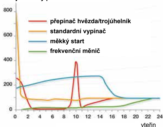
% jmenovitý proud
