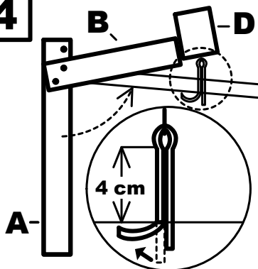
Zahnutí závlačky
