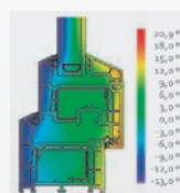
průběh izoterm
