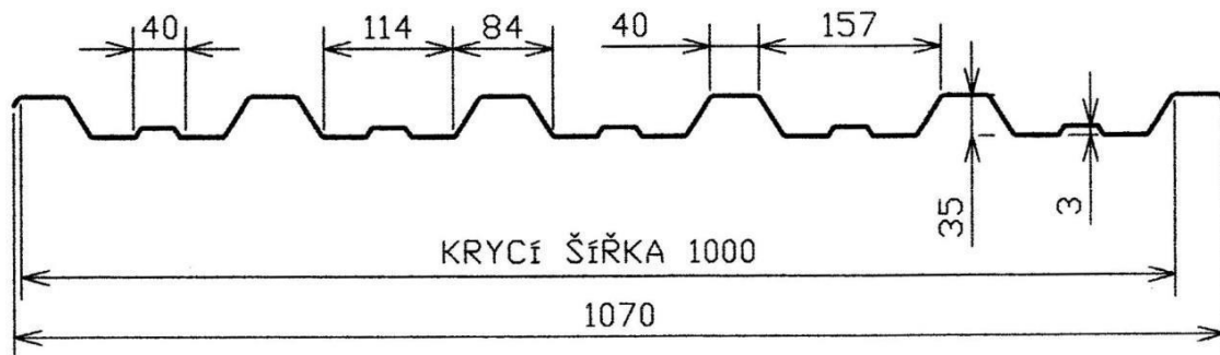
Profil trapézového plechu FERAL 35
