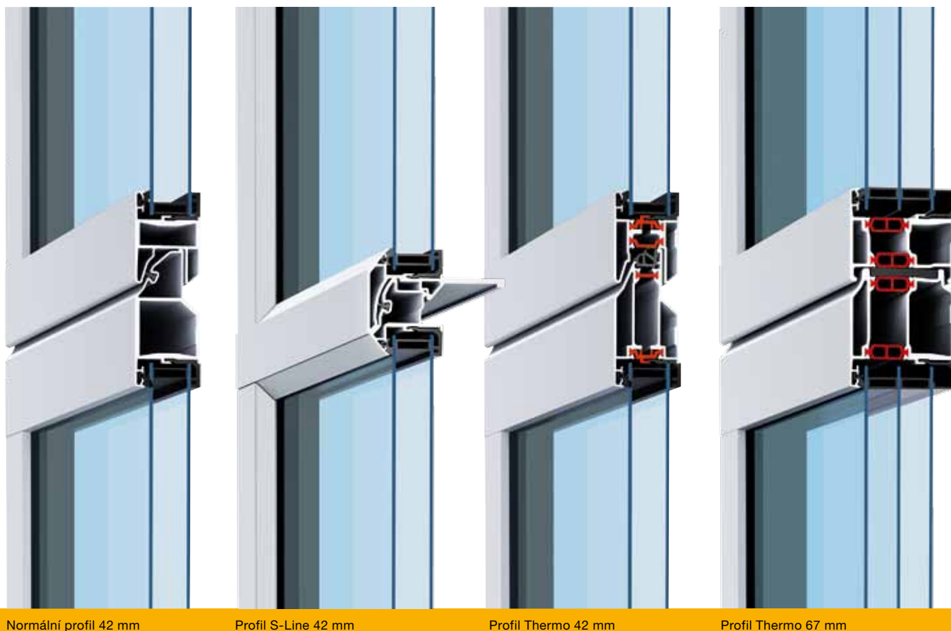
Normální profil 42 mm
