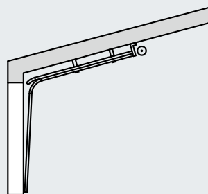
Kování LD* se sklonem podle střechy
