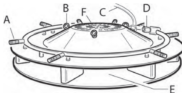
A - trysky/Nozzles B - závěsná oka/chains hooks C - elektrický kabel electric cable D - přívod vody/water inlet E - výstup vzduchu/ air outlet F - vstup vzduchu/air inlet
