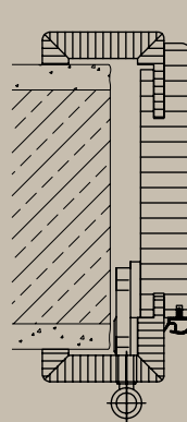
Dřevěná zárubeň, oblá hrana
