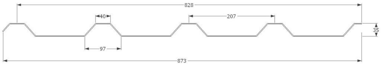
KPTR 35/207 Celková š. 1080 mm Skladební š. 1035 mm
