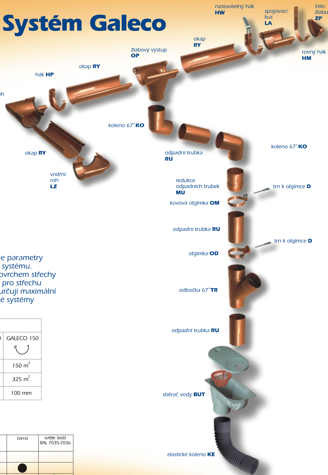
Schéma okapové instalace Galeco 130
