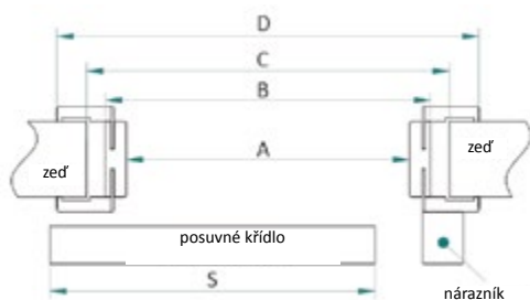
nástěnný posuvný systém se zabudováním
