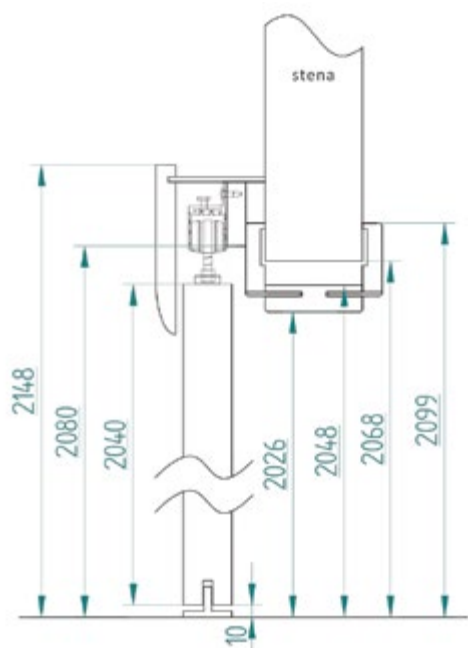
nástěnný posuvný systém se zabudováním
