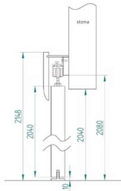
posuvný nástěnný systém bez zabudování
