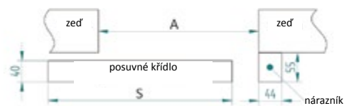
posuvný nástěnný systém bez zabudování
